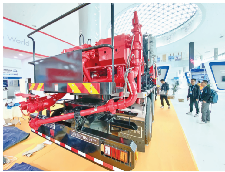
首届四川装备智造国际博览会现场展出的液压传动压裂车
